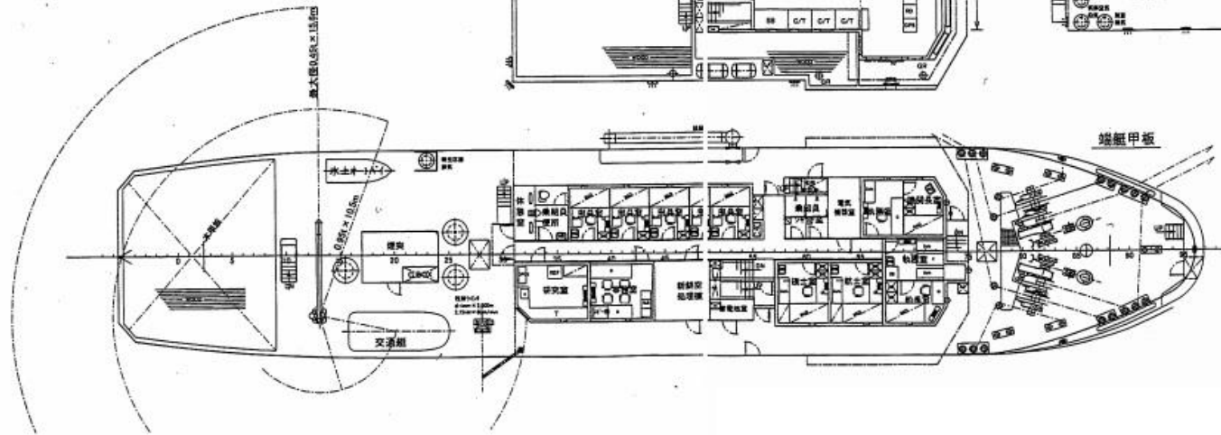
練習船「大島丸」代船 一般配置図 独立行政法人国立高等専門学校機構 大島商船高等専門学校 縮尺 1/200 最終更新日 令和3年5月
